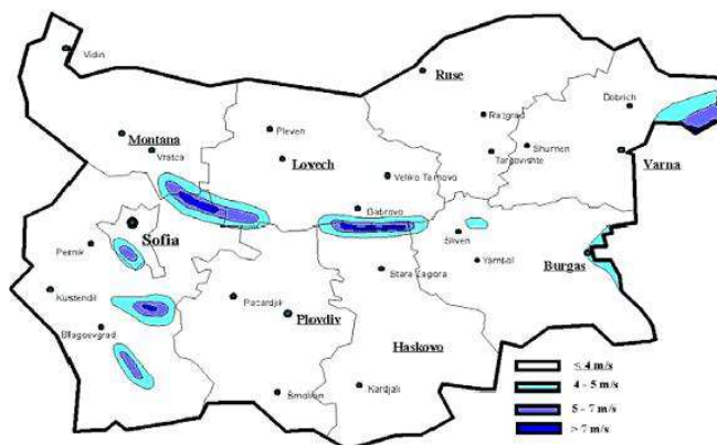
Фиг. 8: Теоретичен потенциал на вятърната енергия в България
